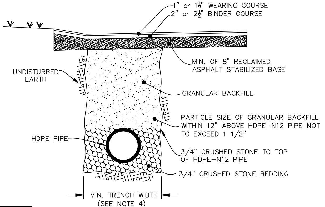
TYPICAL TRENCH CROSS-SECTION (N.T.S.)
